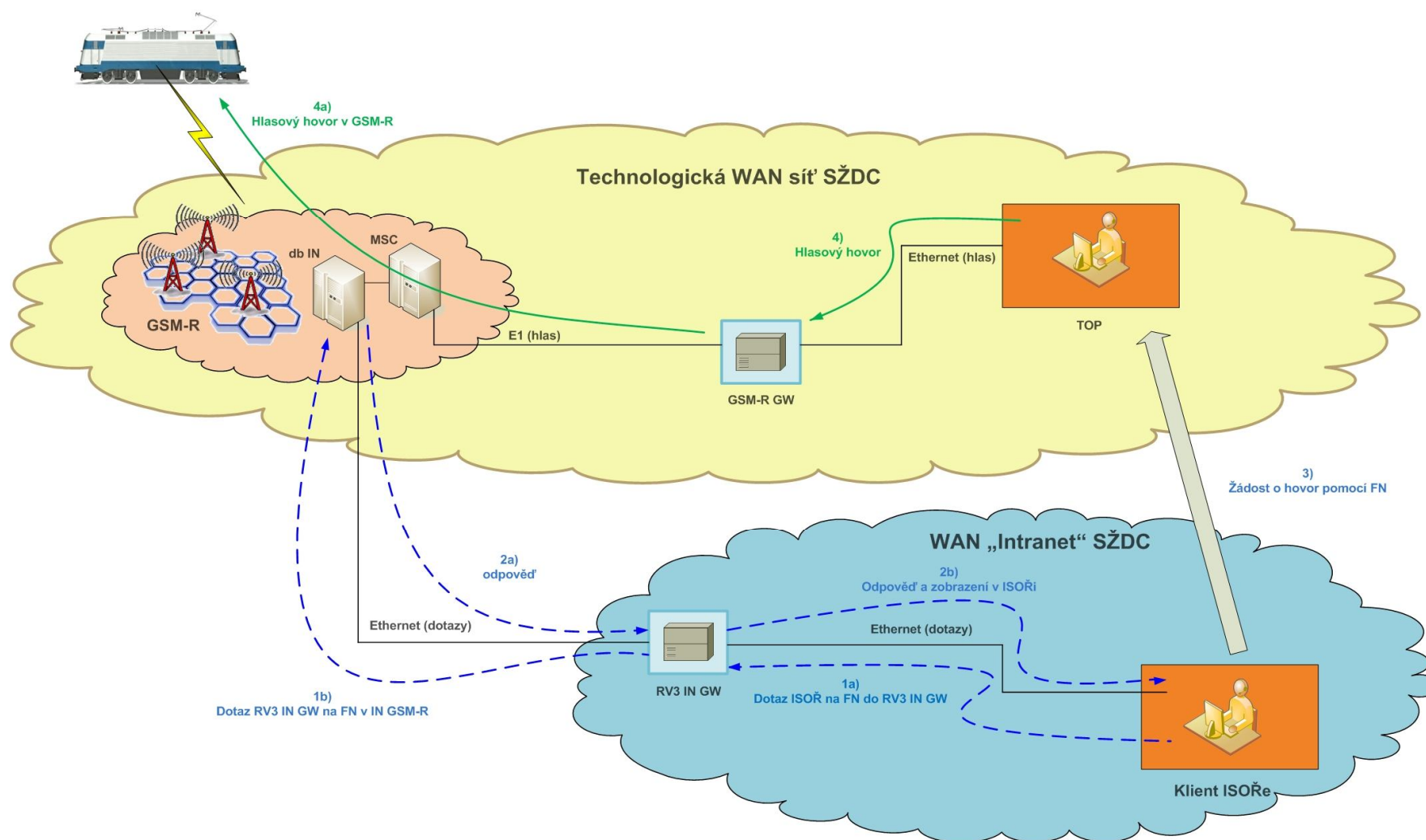
Schéma komunikace klient ISOŘe – RV3 IN GW – db IN a klient ISOŘe – TOP – vlak v GSM-R síti
